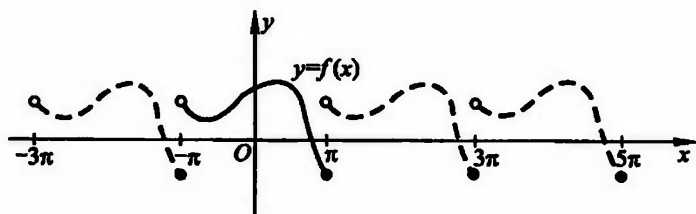
图 15-2 实线与虚线的全体表示 y=f(x)
